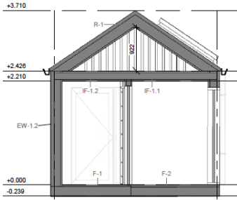
SECTION A-B M 1 : 50
